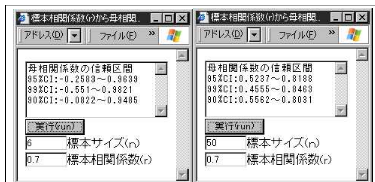
資料 21 山内(1998)の提示した例題( r=0.70 n=6 と n=50 )の実行結果
